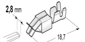
TERMINAL JT FÊMEA 2,8MM FIO 1,5÷2,5
