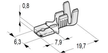
TERMINAL MACHO 6,3MM FIO 1÷2,5
