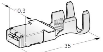
TERMINAL FÊMEA 10,3MM FIO 8÷10
