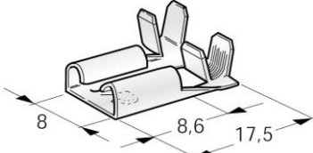
TERMINAL FÊMEA DE FICHA LATERAL 8MM FIO 1÷2,5
