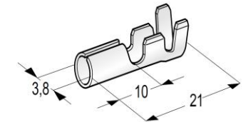
PIN TERMINAL 3,8MM FIO 0,5÷2,5
