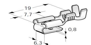
TERMINAL DUPLO 2VIAS 6,3MM FIO 0,8÷2,5
