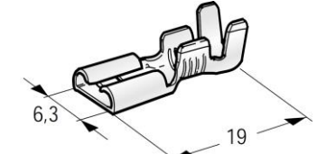
TERMINAL FÊMEA 6,3MM FIO 1÷2,5
