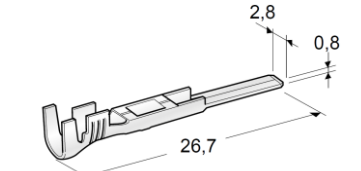
TERMINAL JT MACHO 2,8MM FIO 0,35÷1
