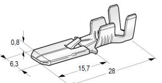
TERMINAL MACHO COM PATILHA DE TRAVÃO 6,3MM FIO 0,75÷2
