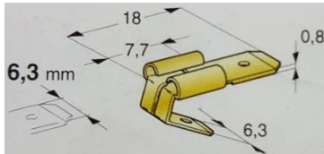
TERMINAL FASTON 3VIAS 6,3MM FIO
