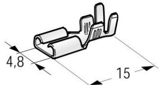
TERMINAL FÊMEA 4,8MM FIO 0,5÷1
