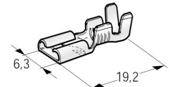
TERMINAL FÊMEA COM PATILHA DE TRAVÃO 6,3MM FIO 1÷2,5
