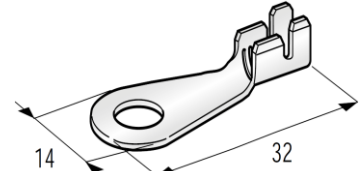
TERMINAL OLHAL M6 MACHO FIO 8÷10
