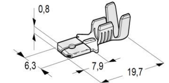
TERMINAL MACHO 6,3MM FIO 0,5÷1
