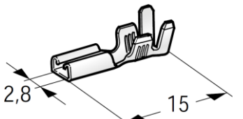
TERMINAL FÊMEA 2,8MM FIO 0,3÷1
