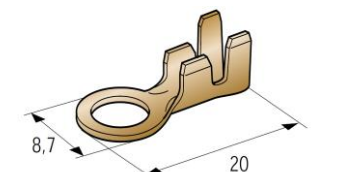
TERMINAL DE OLHAL M5 8,7MM FIO 1÷2,5
