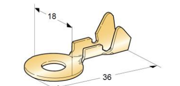
TERMINAL DE OLHAL M10 FIO 4÷6
