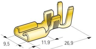
TERMINAL FÊMEA 9,5MM FIO 3÷6
