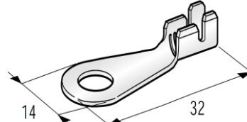
TERMINAL OLHAL M6 MACHO FIO 4÷6
