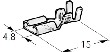
TERMINAL FÊMEA COM TRAVAO 4,8MM FIO 0,5÷1
